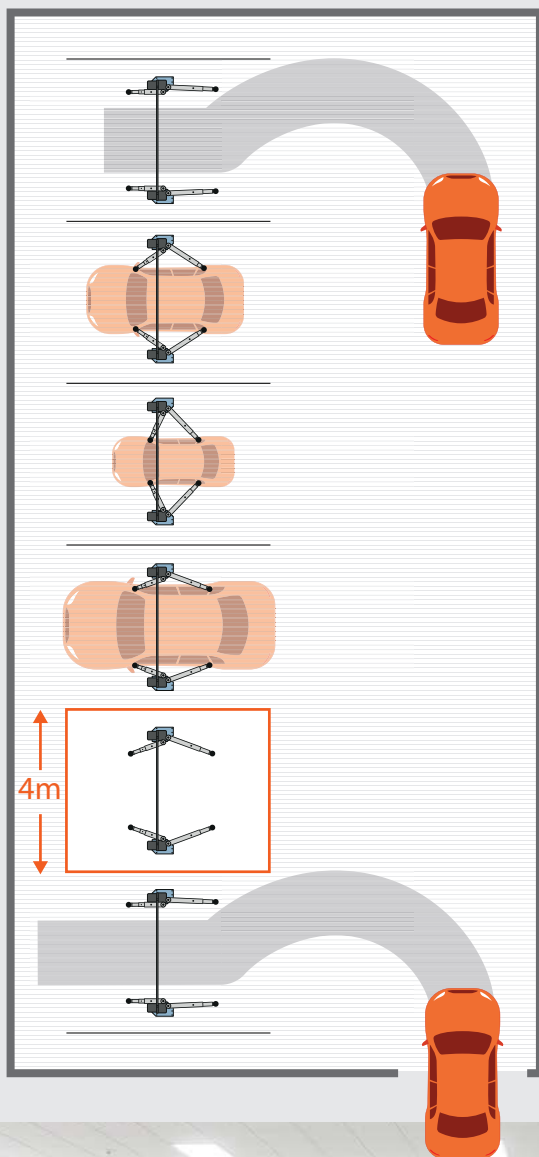
Podnośnik dwukolumnowy
